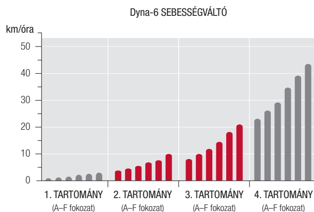
SZÁNTÓFÖLDI MUNKAVÉGZÉS SEBESSÉGTARTOMÁNYA
