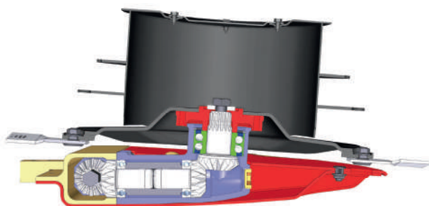
A kaszagerendely keresztmetszete
